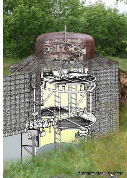
Fotomontasje av kuppelen til R633. Her ser vi at bygningen har flere etager og inneholder mye mekanik. Fotomontasjon/ Tegningen er laget av Jurga.
